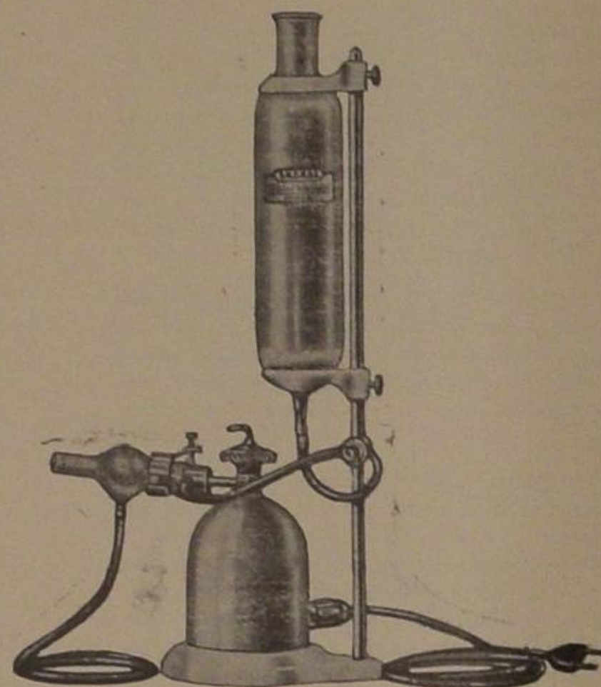
Inalatore OMCROS a vapore per acque termali Mod. A. T. da tavolo
